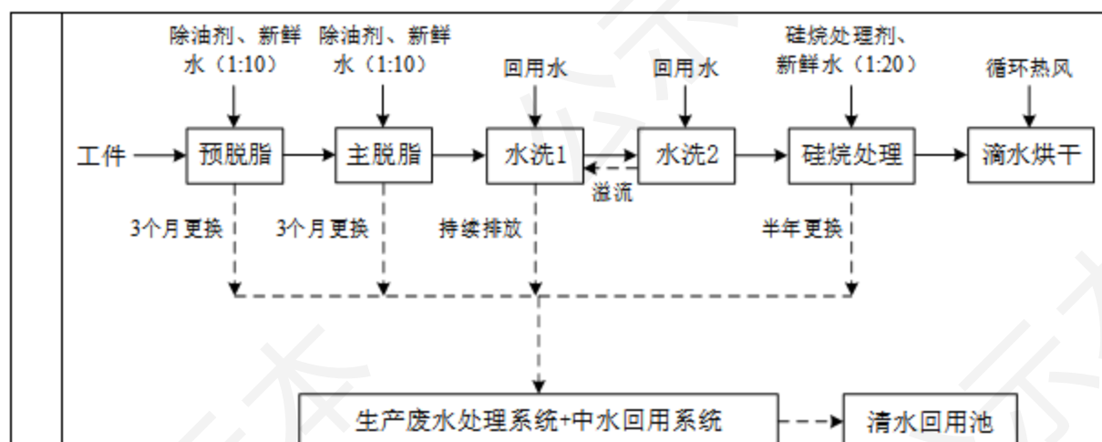
图2-5 前处理线生产工艺流程图
