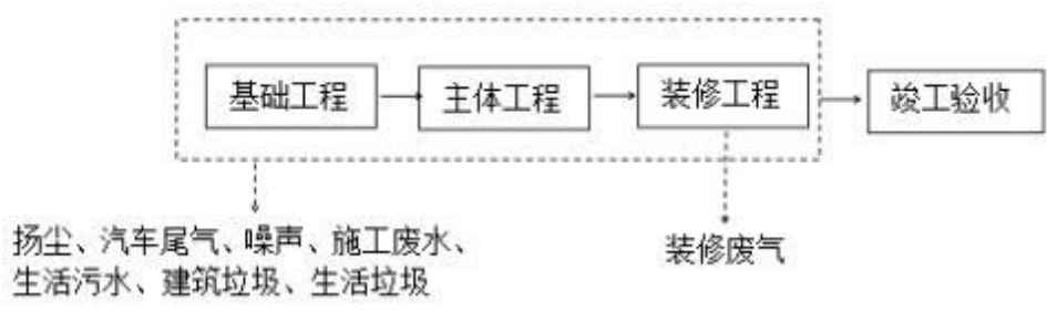
图 2-3 本项目施工期工艺流程及产污环节图
