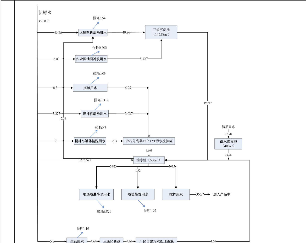
图 2-2 项目降雨期间水平衡图 (t/d)
