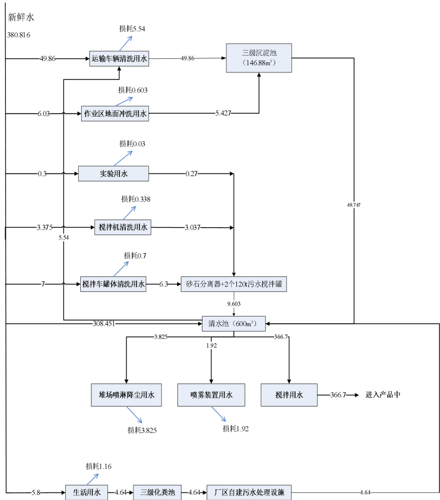
图 2-1 项目非降雨期水平衡图 (t/d)
