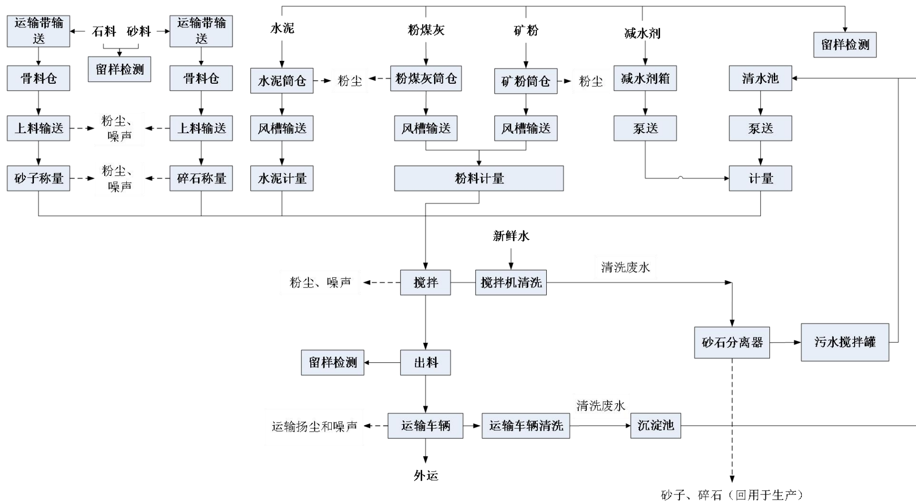
图 2-5 项目混凝土生产工艺流程及产污环节示意图
