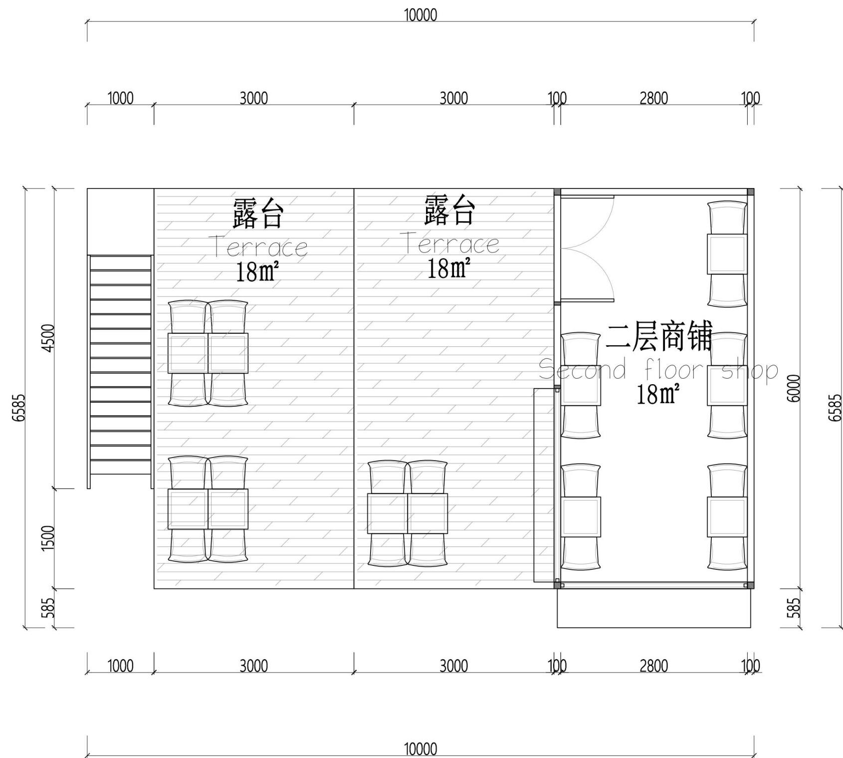
双层集装箱样式1-2层平面图
