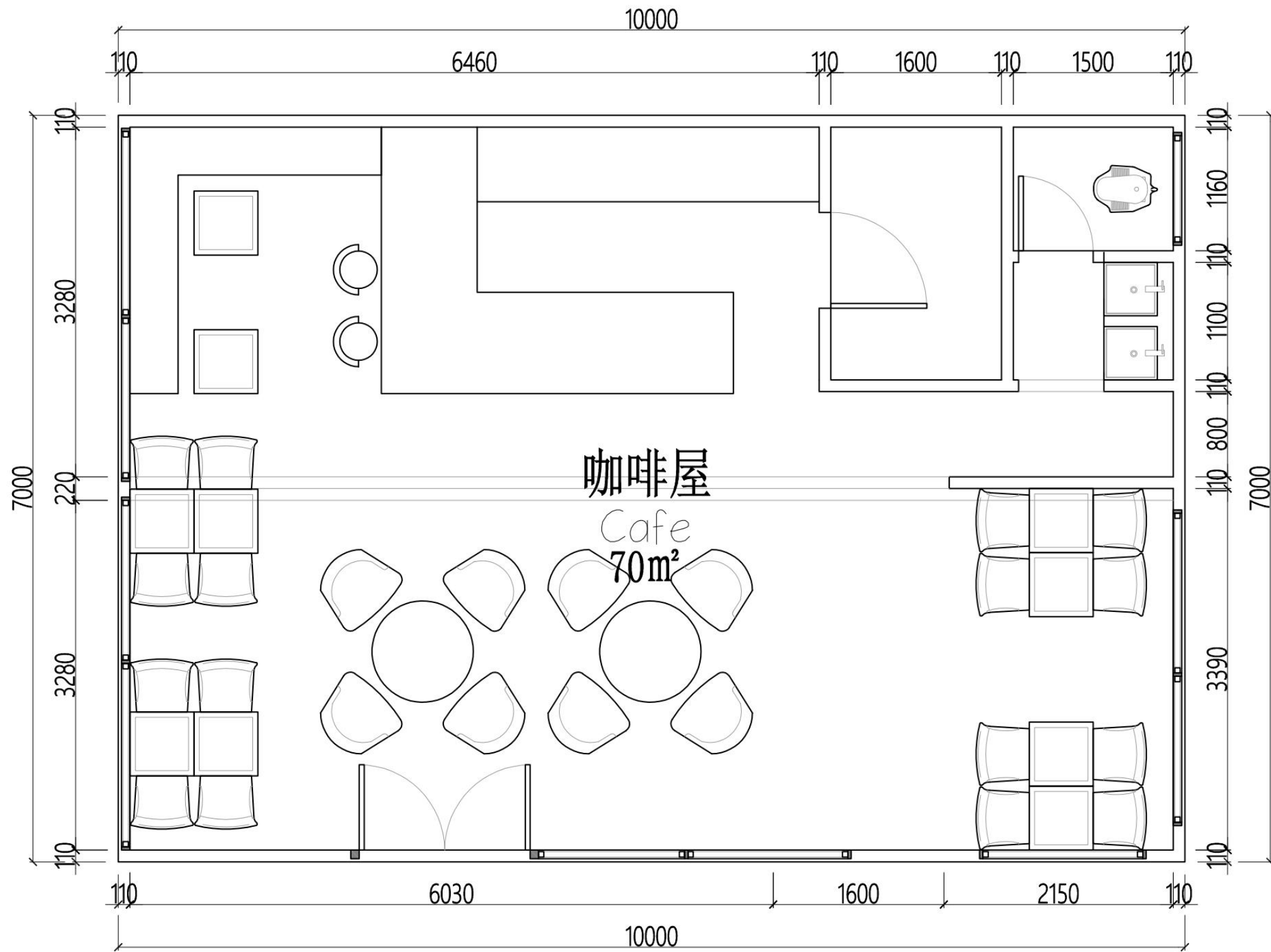
咖啡屋一平面图
